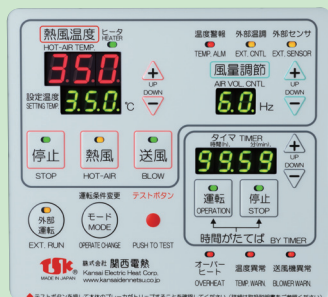
操作パネル
