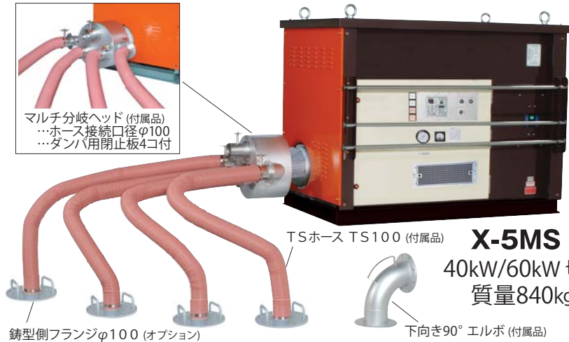
鑄型側フランジφ100 (オプション)
