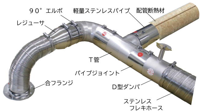
< 配管施工例 > … 接ガス部はオールSUS
